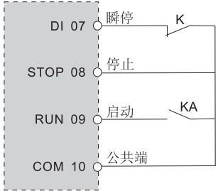
继电器控制方式
