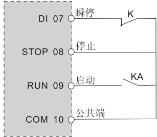
异地控制方式
